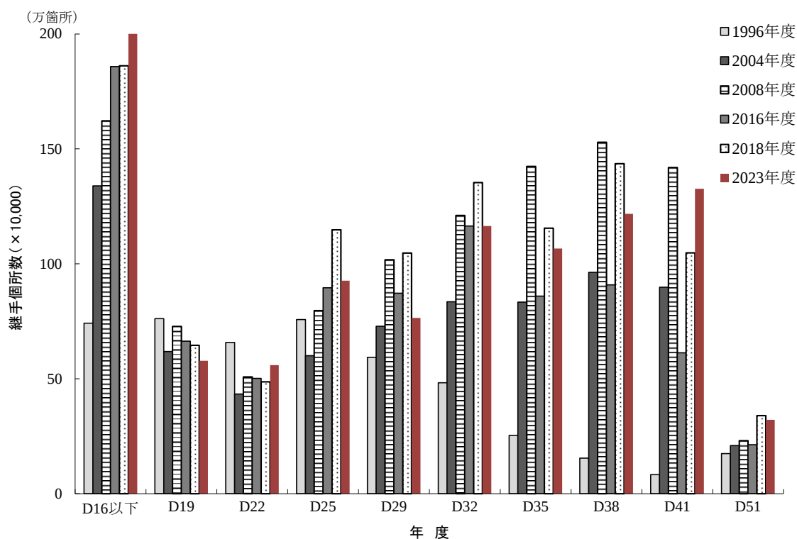
図 3.9 機械式継手の鉄筋径別・年度別の施工実績
