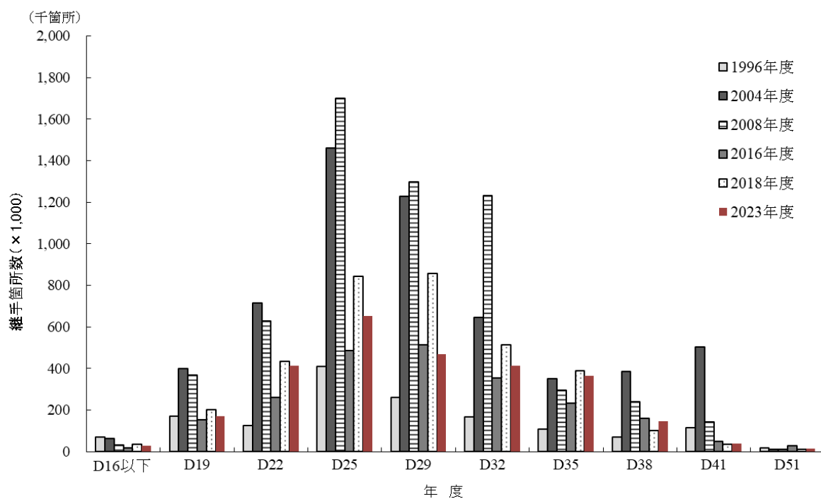
図 3.11 溶接継手の鉄筋径別・年度別の施工実績
