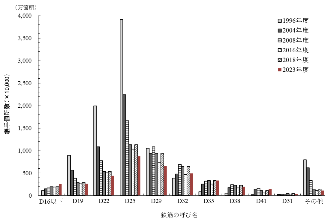
図 3.6 鉄筋継手全体の鉄筋径別・年度別の施工実績
