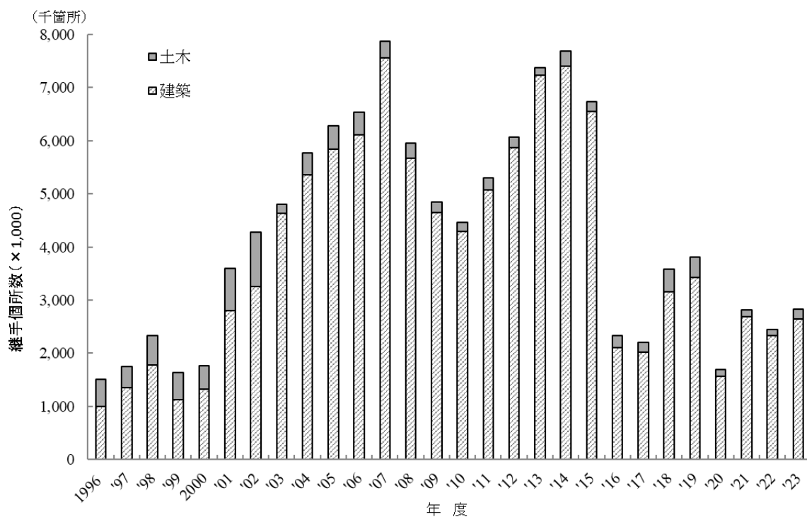
図 3.12 溶接継手の工事分野別の施工実績
