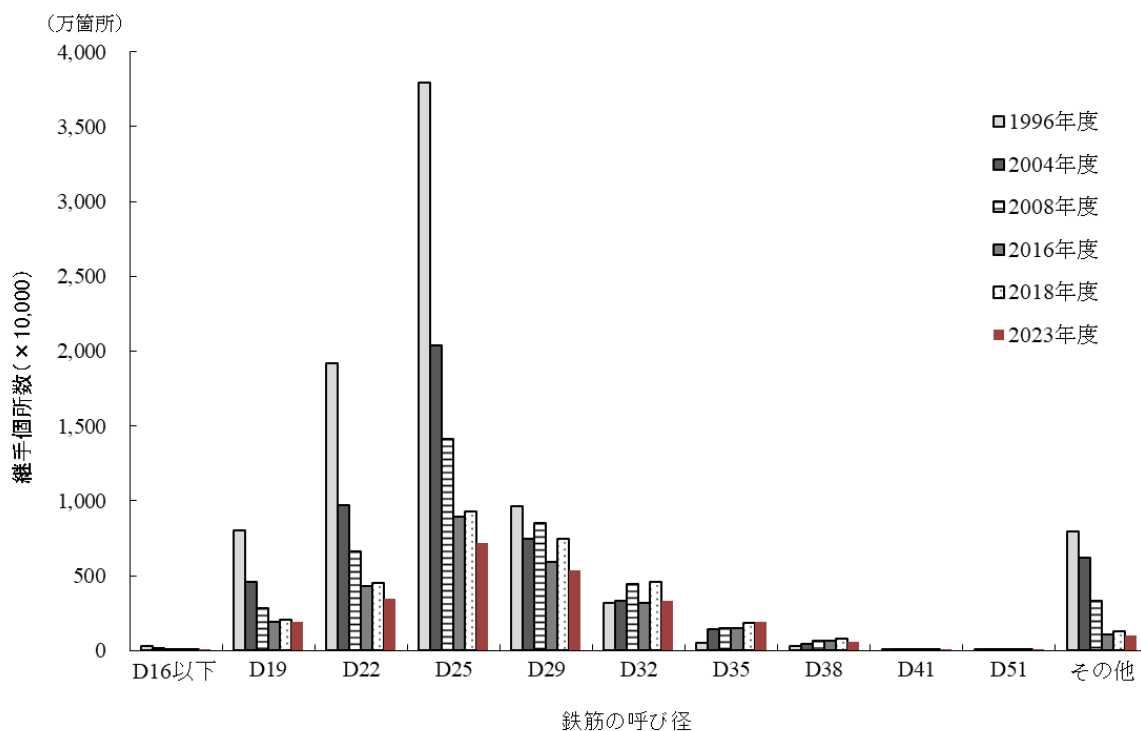
図 3.7 ガス圧接継手の鉄筋径別・年度別の施工実績
