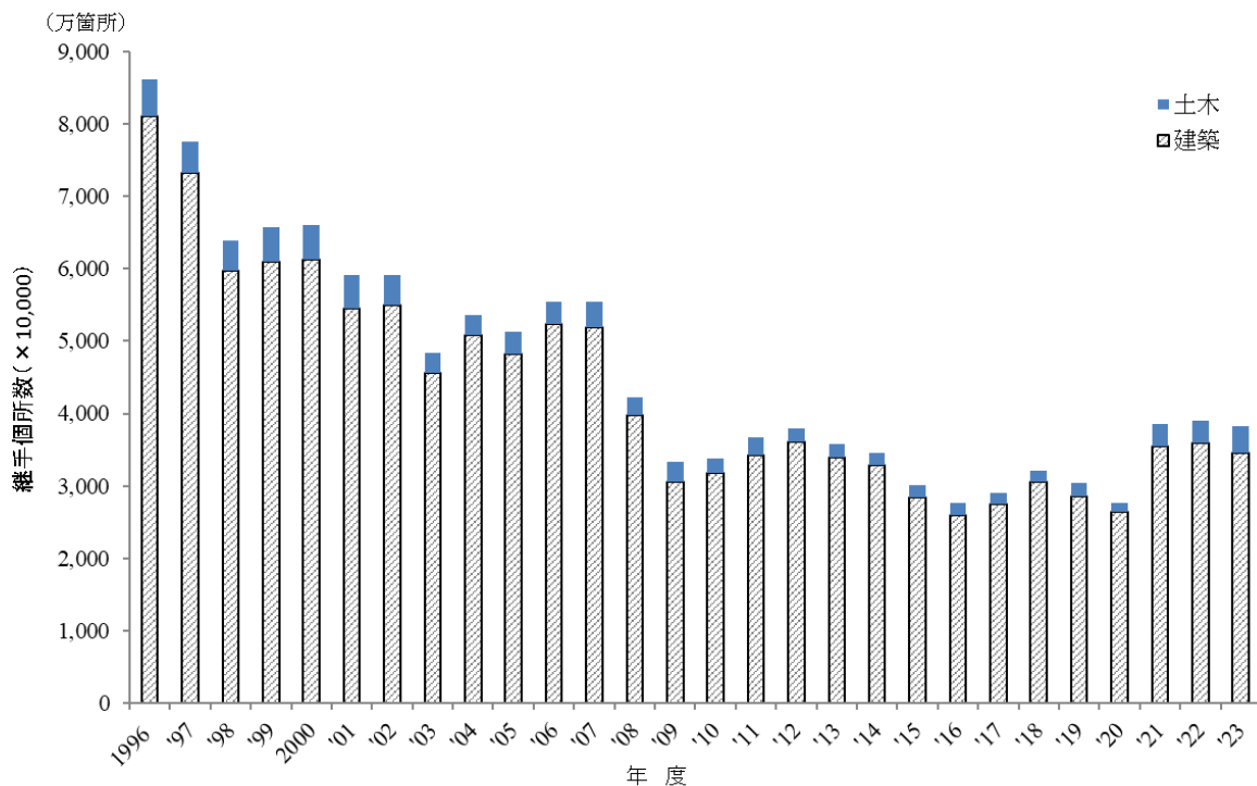
図 3.8 ガス圧接継手の工事分野別の施工実績
