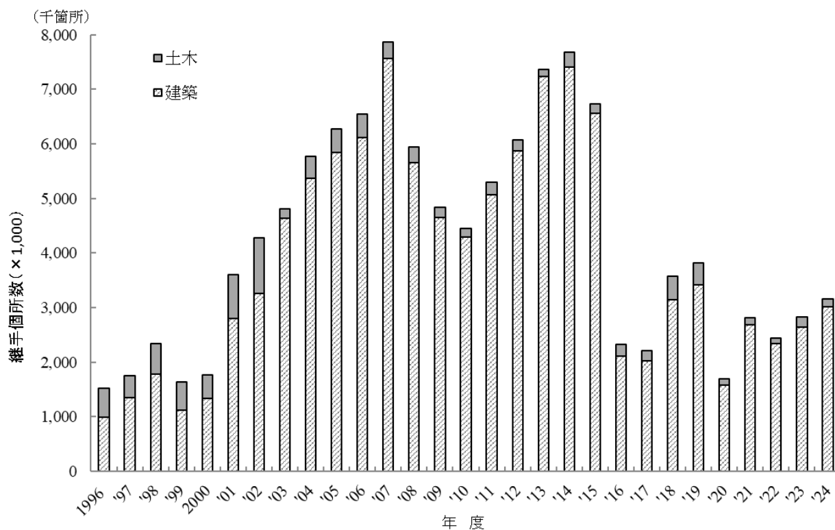
図 3.12 溶接継手の工事分野別の施工実績
