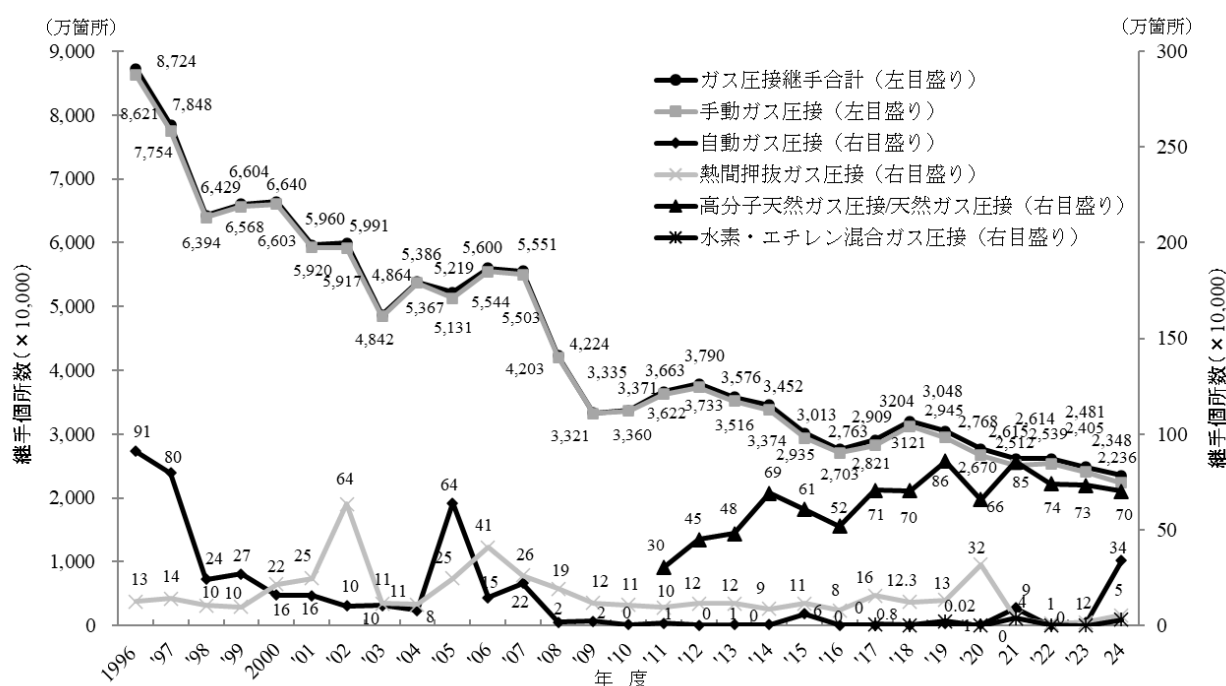
図 3.2 ガス圧接継手の工法別の施工実績推移
