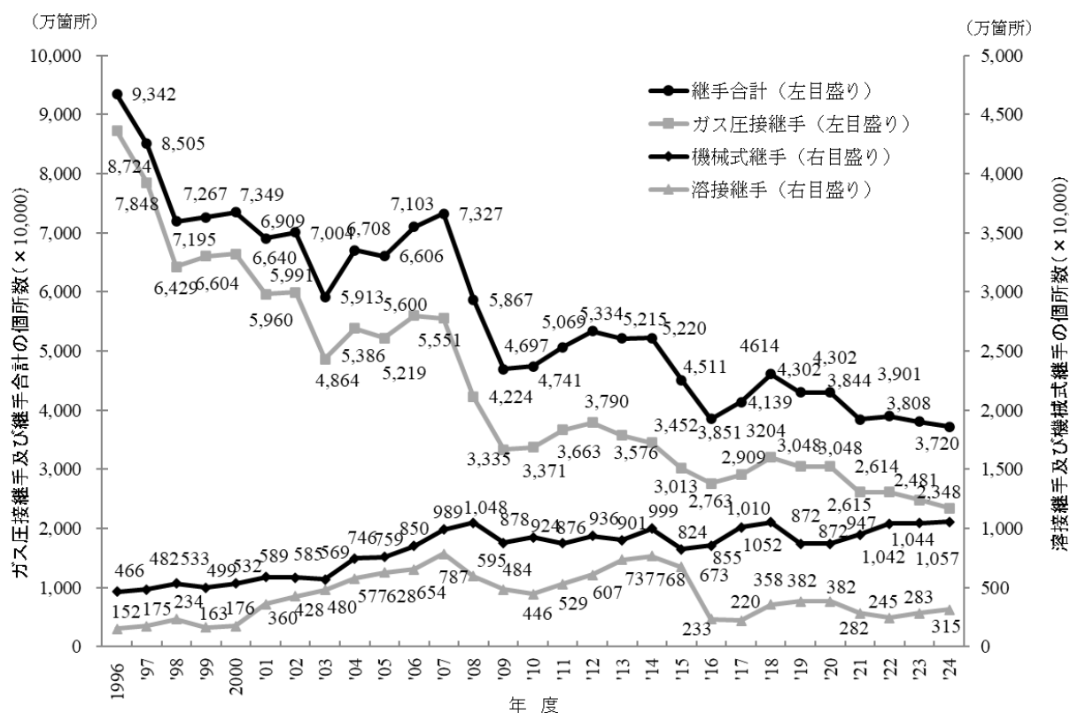
図 3.1 鉄筋継手工法別の施工実績推移
