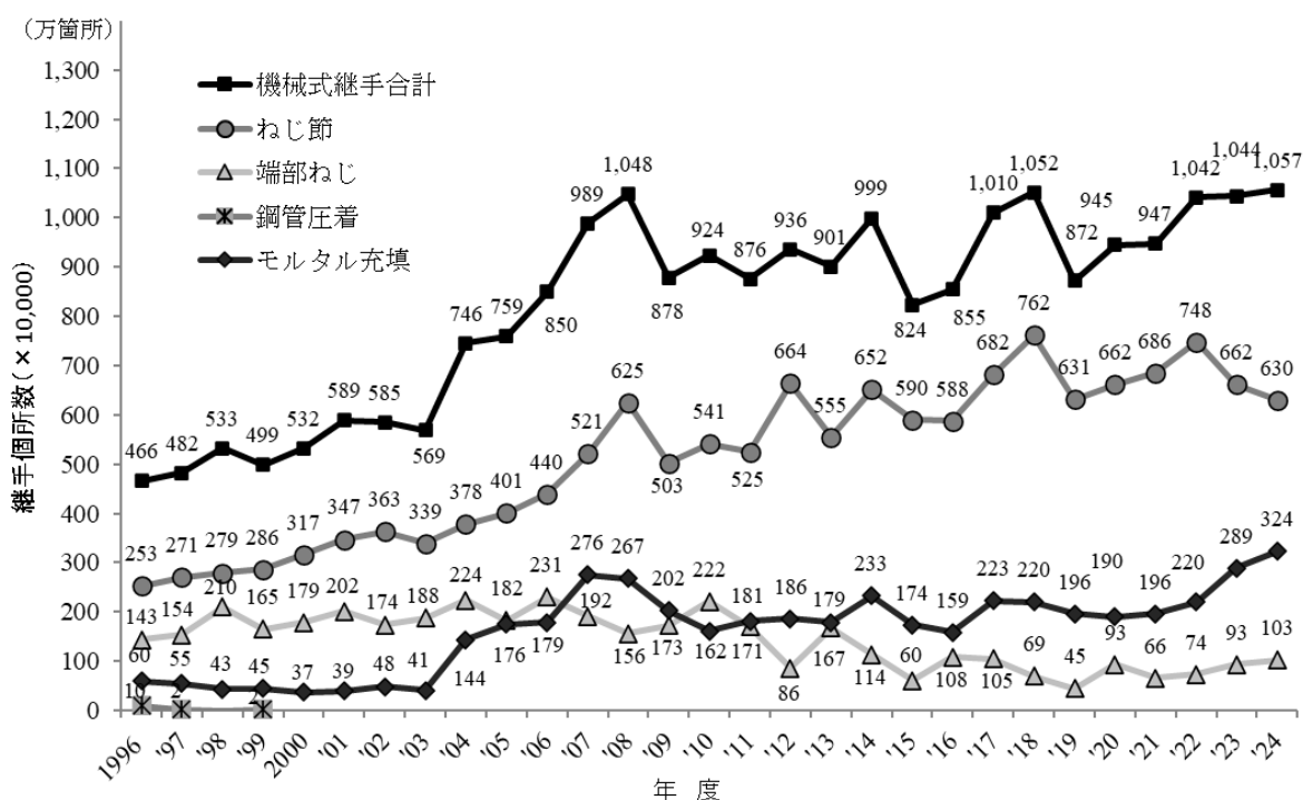
図 3.3 機械式継手の工法別の施工実績推移
