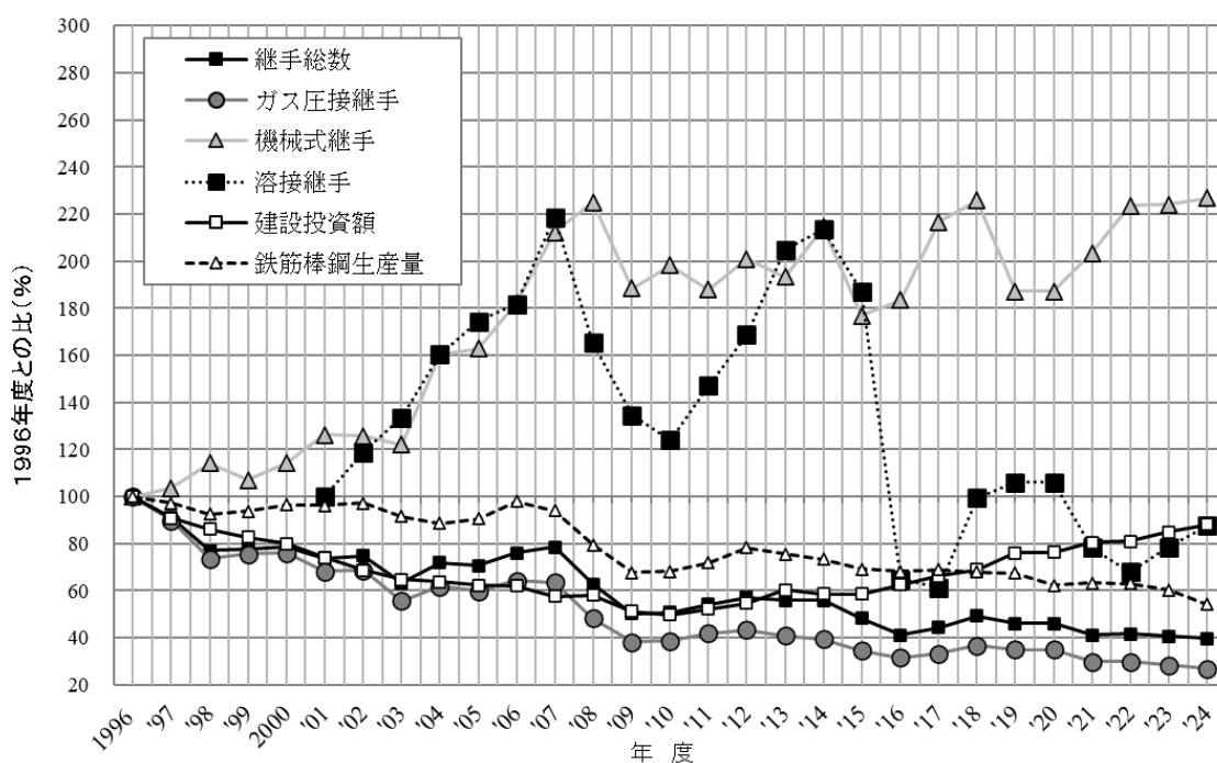
図 3.5 各年度の施工実績の1996年度に対する増減率
