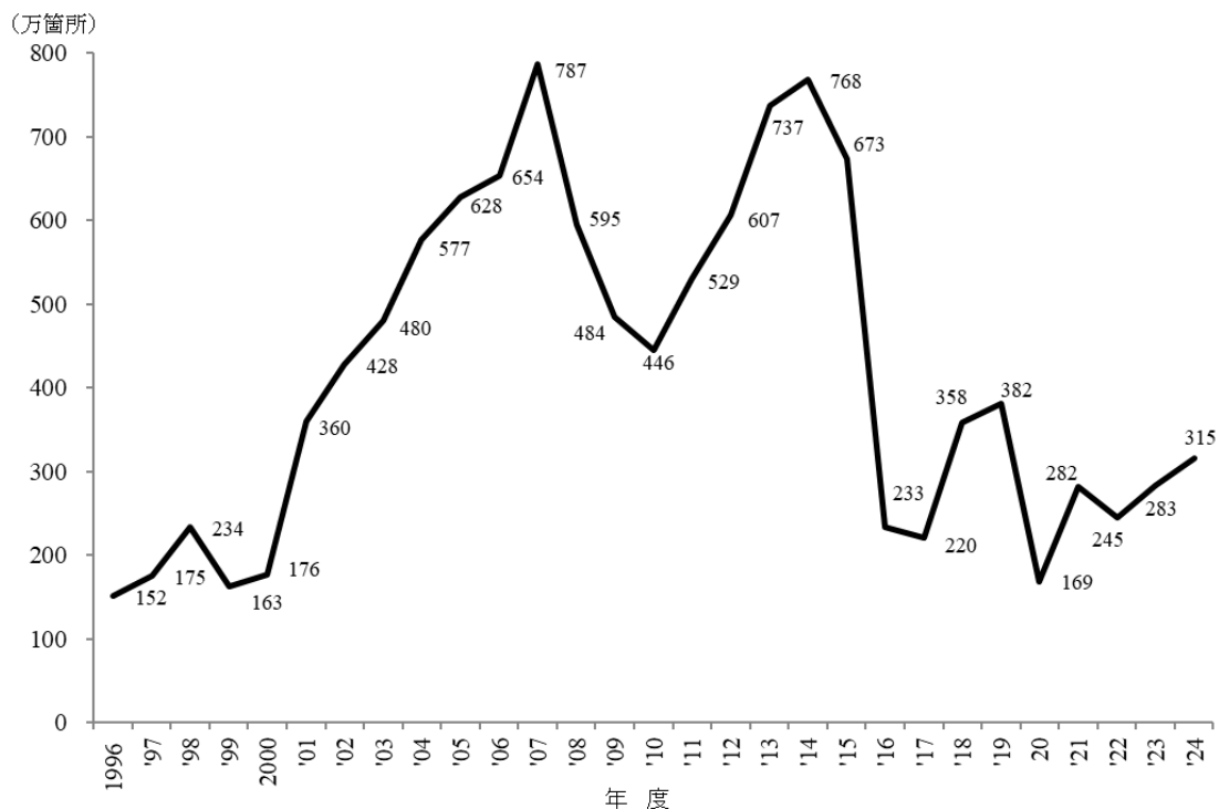
図 3.4 溶接継手の施工実績推移
