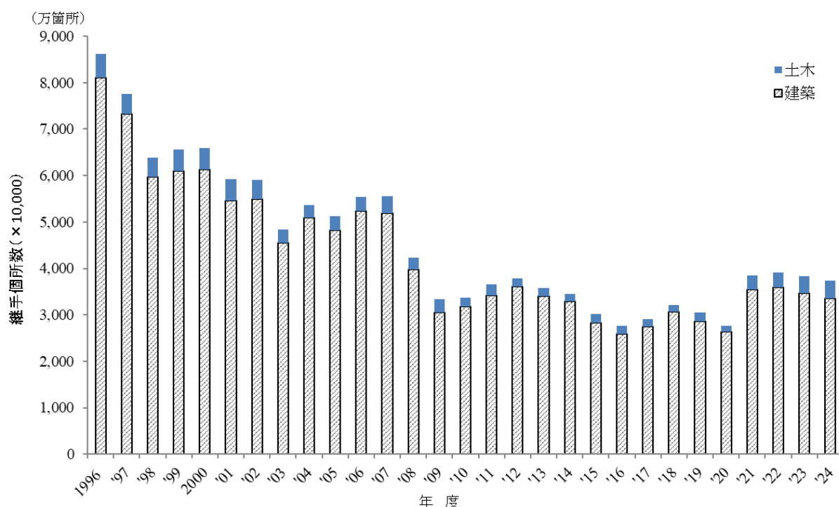
図 3.8 ガス圧接継手の工事分野別の施工実績
