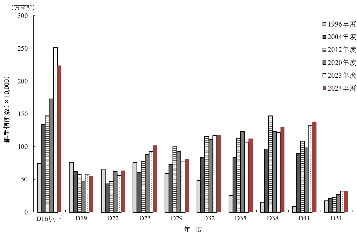
図 3.9 機械式継手の鉄筋径別・年度別の施工実績
