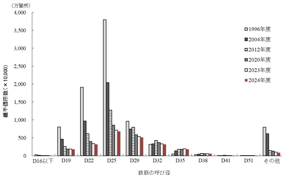
図 3.7 ガス圧接継手の鉄筋径別・年度別の施工実績
