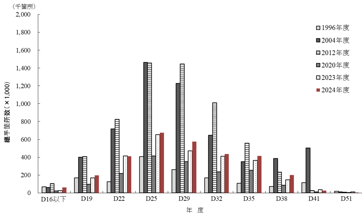
図 3.11 溶接継手の鉄筋径別・年度別の施工実績
