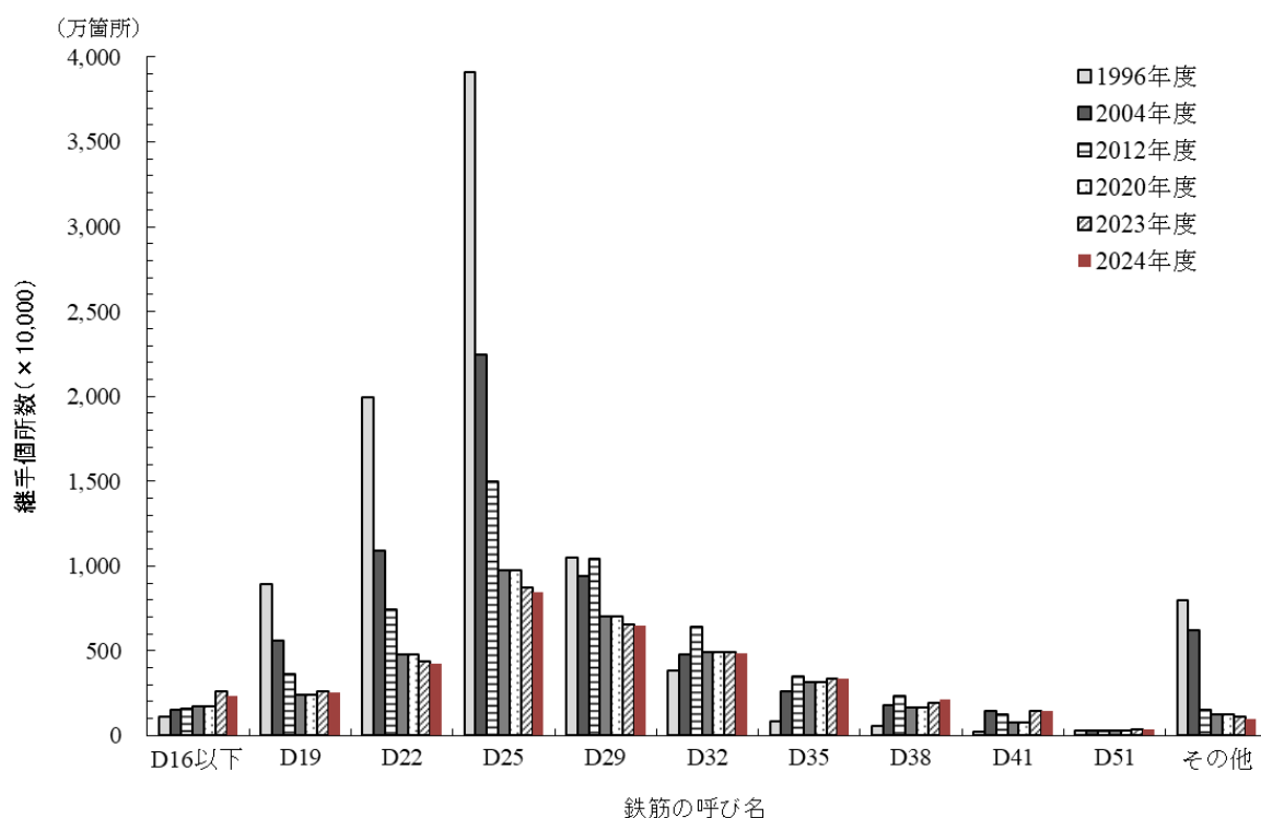
図 3.6 鉄筋継手全体の鉄筋径別・年度別の施工実績
