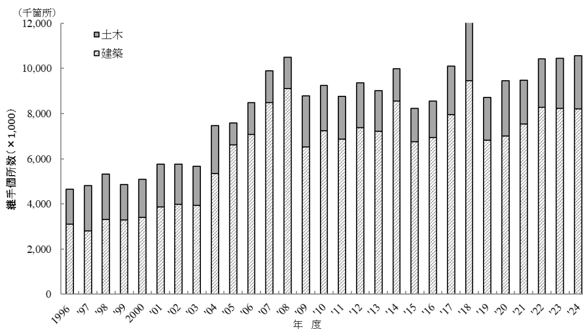
図 3.10 機械式継手の工事分野別の施工実績
